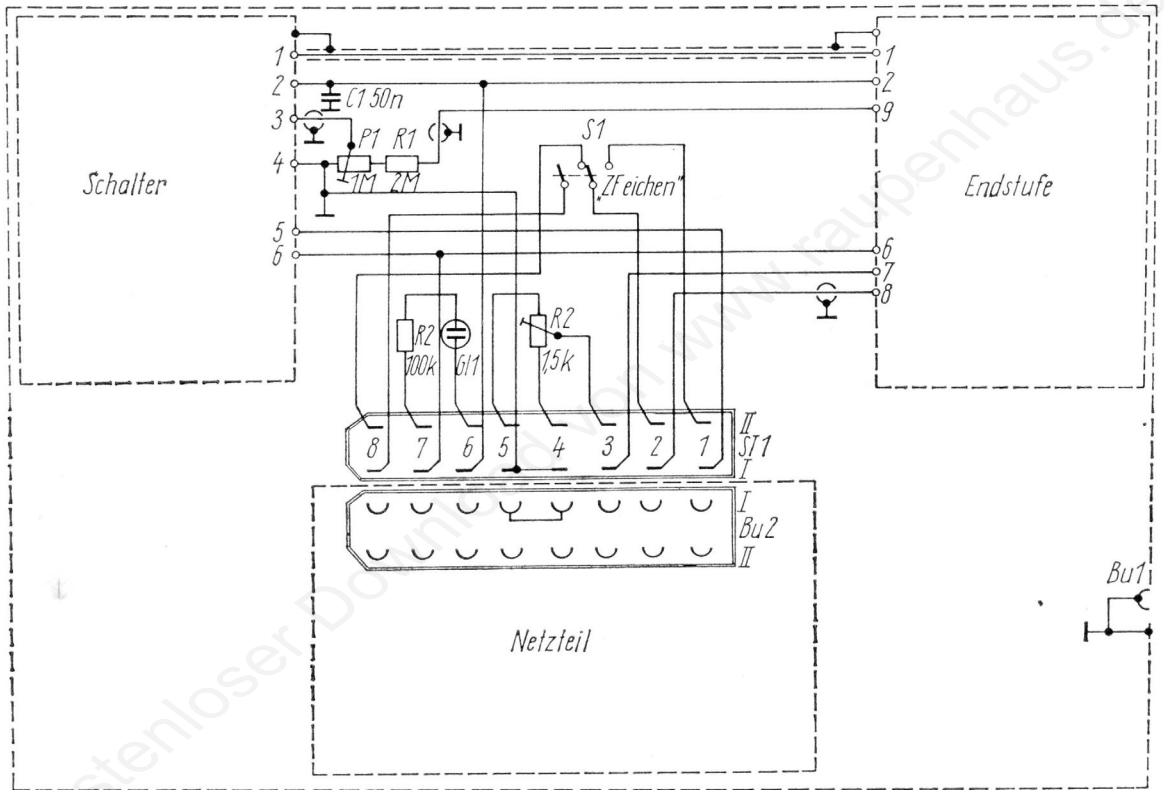
Prüfgenerator PG 2 - Übersicht
