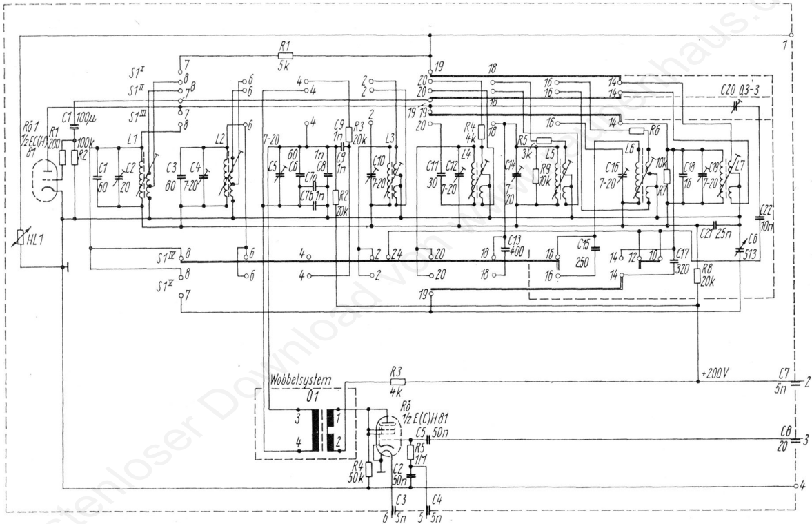
Prüfgenerator PG 2 - Baugruppe Schalter
